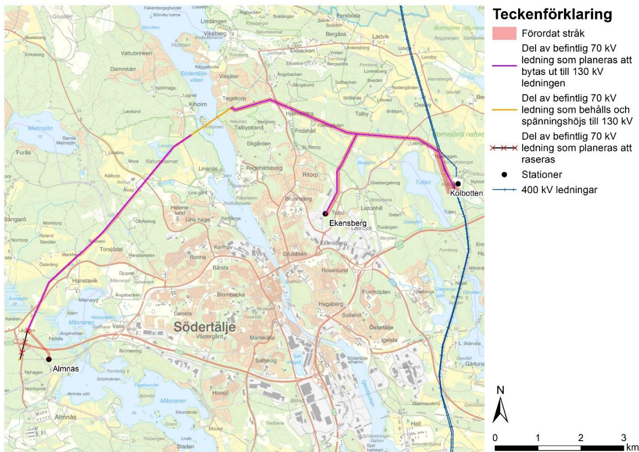
Figur 11. Översikt över delar av befintlig 70 kV ledning som planeras att raderas, bytas ut eller stå kvar.
